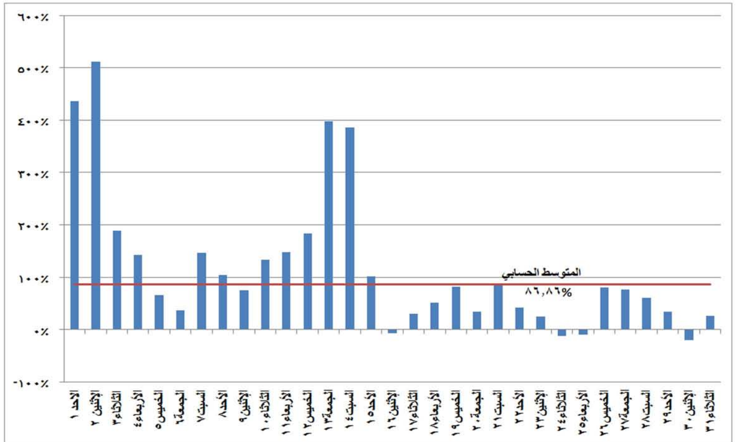
شكل (٢٥) الطاقة الكهربائية المنتجة من الرياح والشمس خلال شهر يوليو ٢٠١٨
