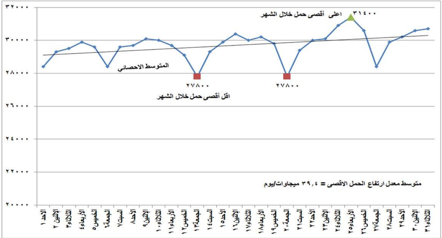
شكل (١) تطور الحمل الاقصى اليومي خلال شهر يوليو ٢٠١٨
