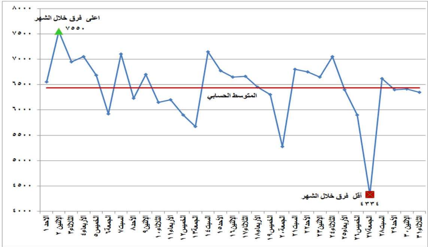
شكل (٣) الفرق بين أقصى وأدنى حمل خلال شهر يوليو ٢٠١٨
