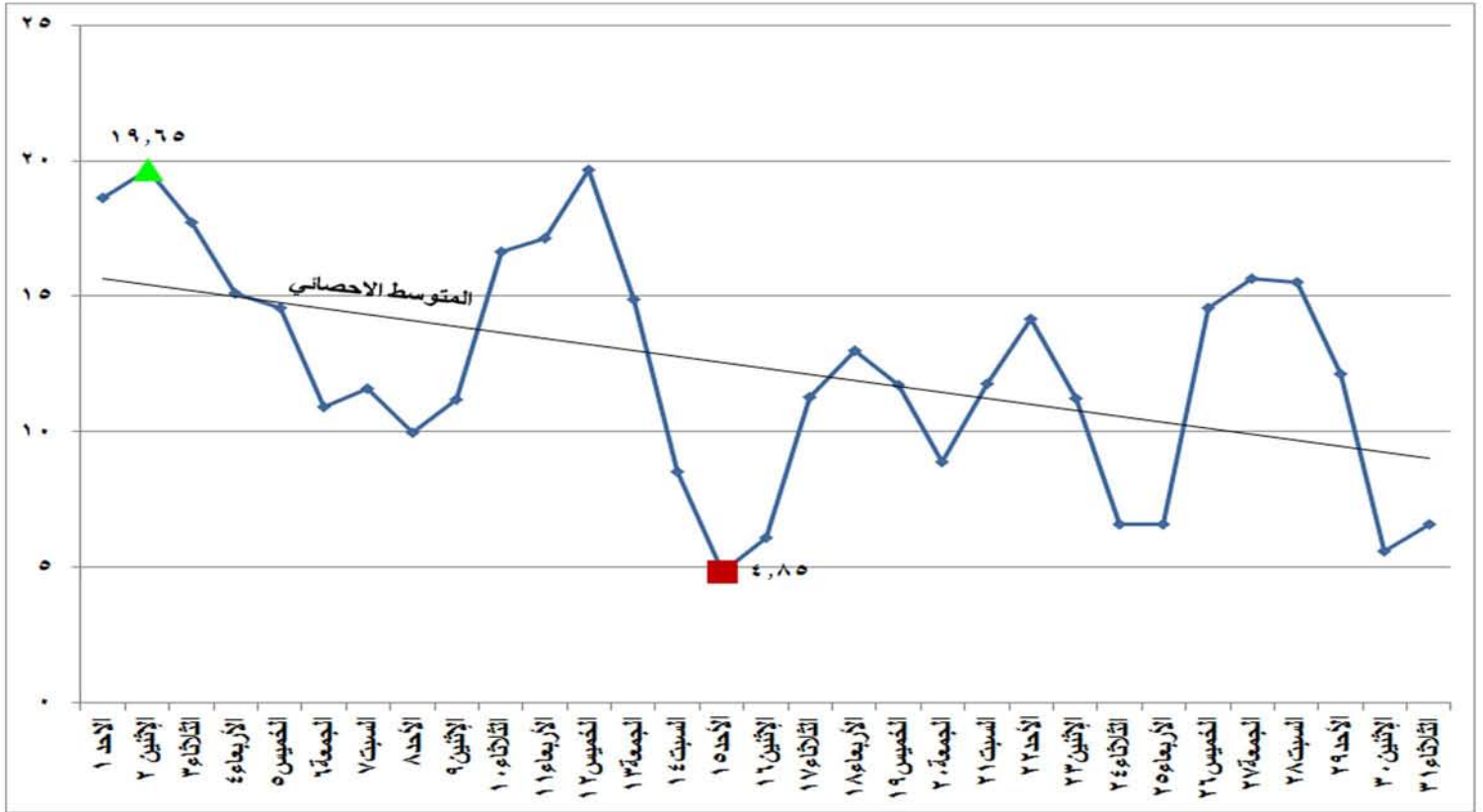
شكل (٢٥) الطاقة الكهربائية المنتجة من الرياح والشمس خلال شهر يوليو ٢٠١٨
