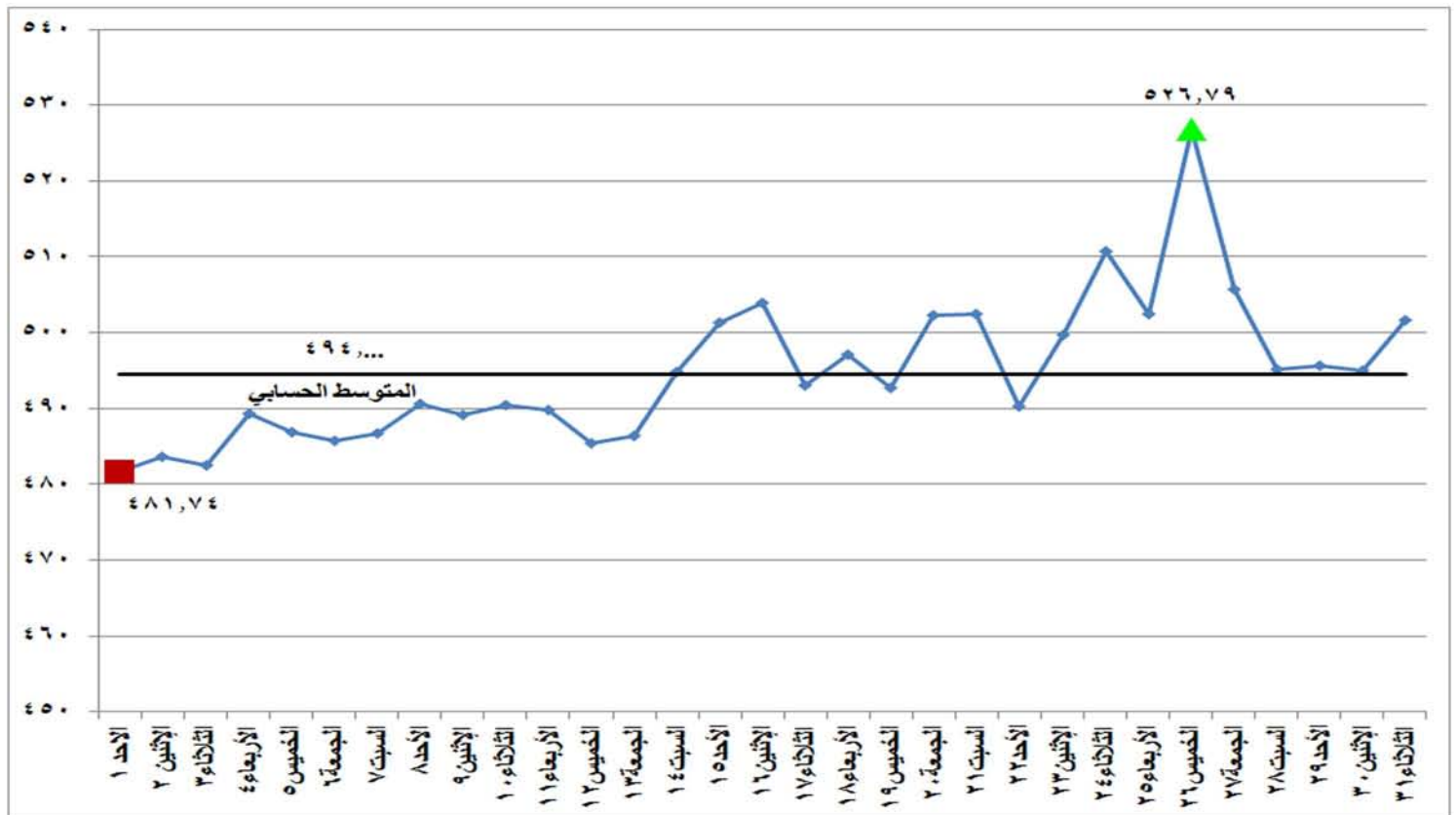
شكل (١٤) معامل انبعاثات غاز ثاني اكسيد الكربون المكافئ على مدى شهر يوليو ٢٠١٨
