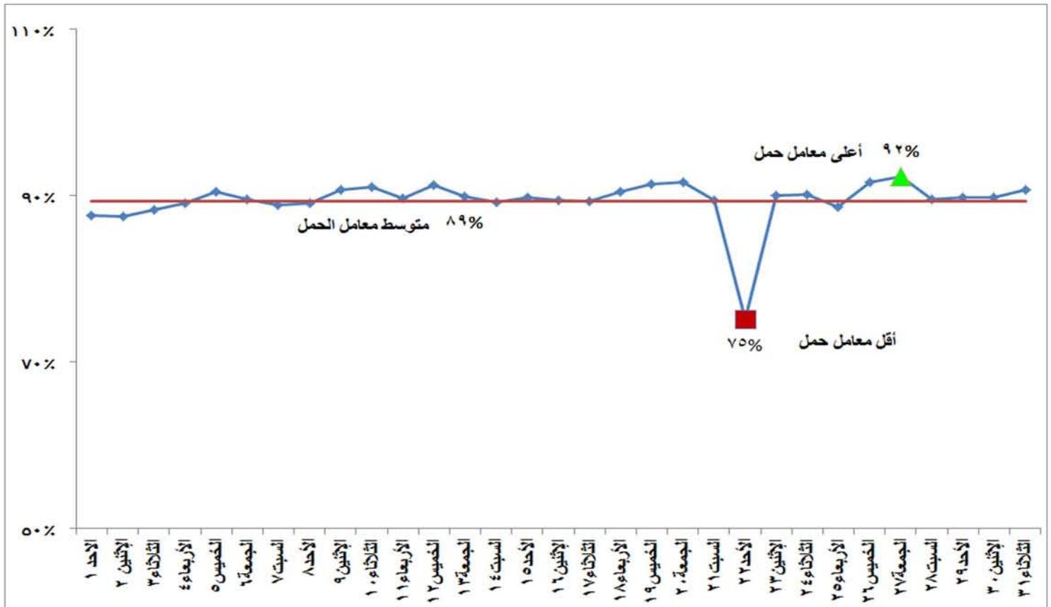
شكل (١٢) إجمالي معامل الحمل لوحدات الانتاج خلال شهر يوليو ٢٠١٨
