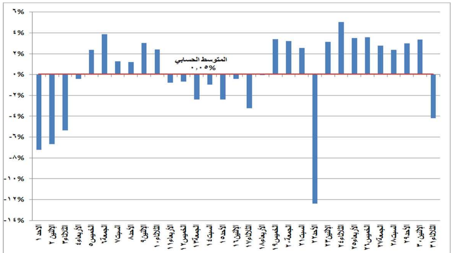
شكل (١٦) نسب التغير في الطاقة الكهربائية المنتجة خلال شهر يوليو ٢٠١٨ مقارنة بالشهر المماثل من العام السابق
