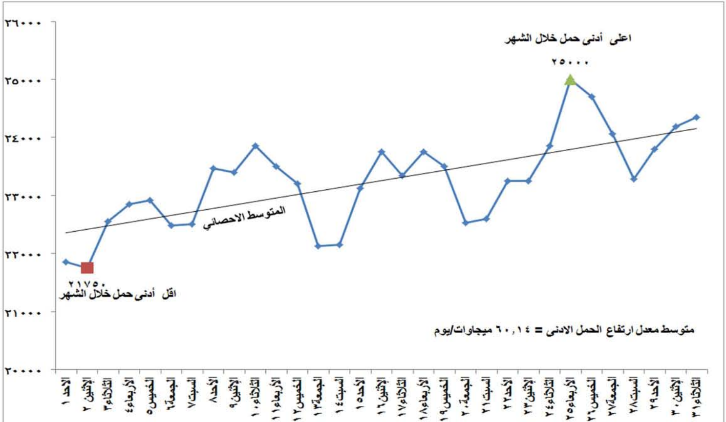
شكل (٢) تطور الحمل الادنى اليومي خلال شهر يوليو ٢٠١٨
