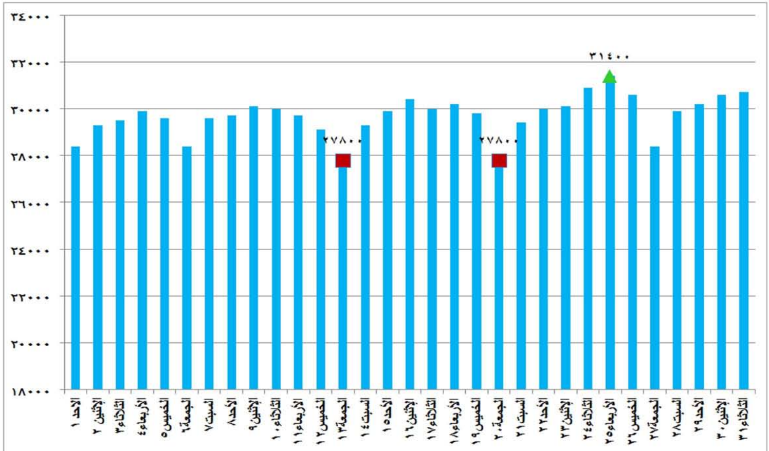
شكل (٥) قدرات الانتاج المتاحة ونسبتها للحمل الأقصى خلال شهر يوليو ٢٠١٨
