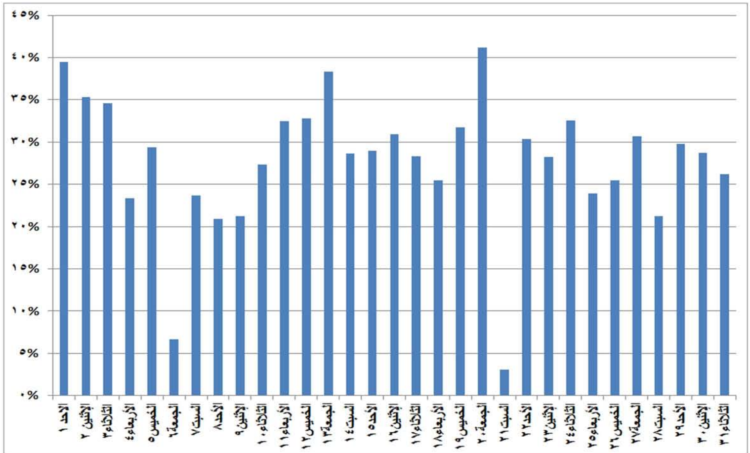
شكل (٢٨) نسب الفائض للحمل الاقصى المسجل يوميا خلال شهر يوليو ٢٠١٨
