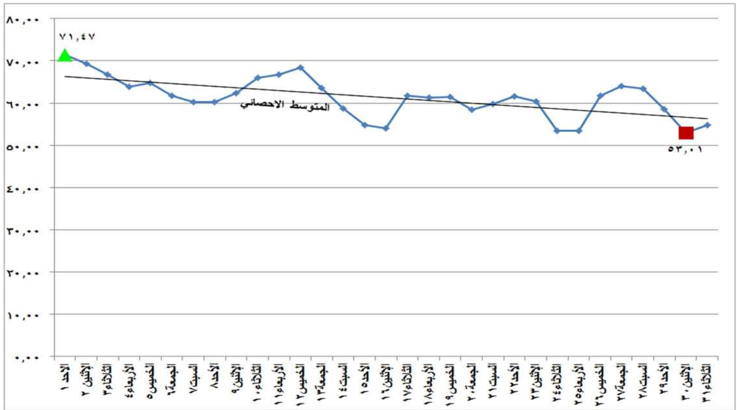
شكل (٢١) الطاقة الكهربائية المنتجة من المصادر غير الحرارية خلال شهر يوليو ٢٠١٨
