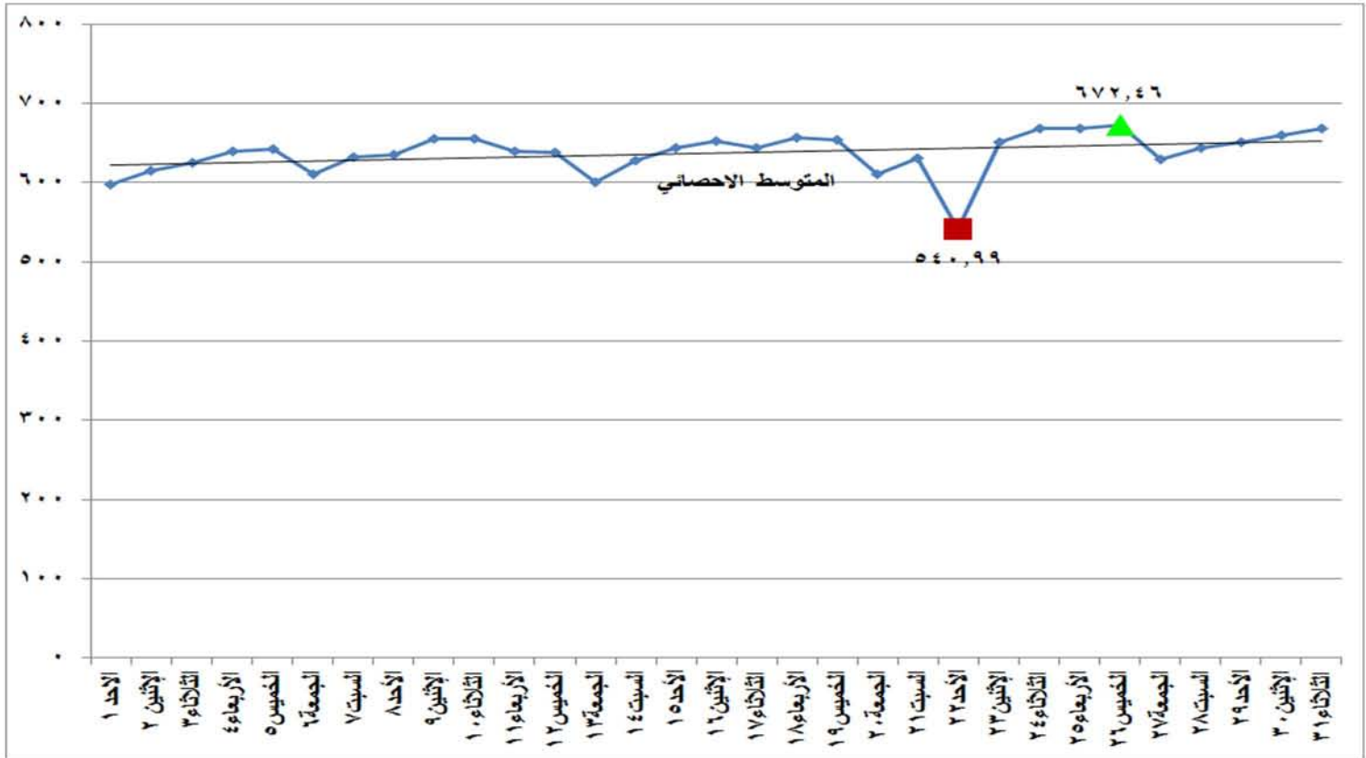
شكل (١٥) إجمالي الطاقة الكهربائية المنتجة من كل المصادر الأولية خلال شهر يوليو ٢٠١٨
