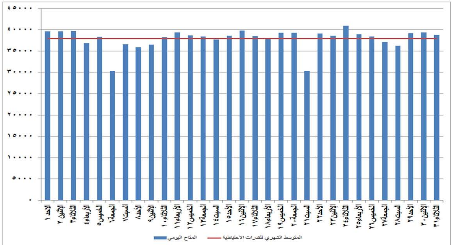
شكل (٢٧) القدرات المتاحة يوميا والمتوسط الشهري للقدرة الاحتياطية خلال شهر يوليو ٢٠١٨
