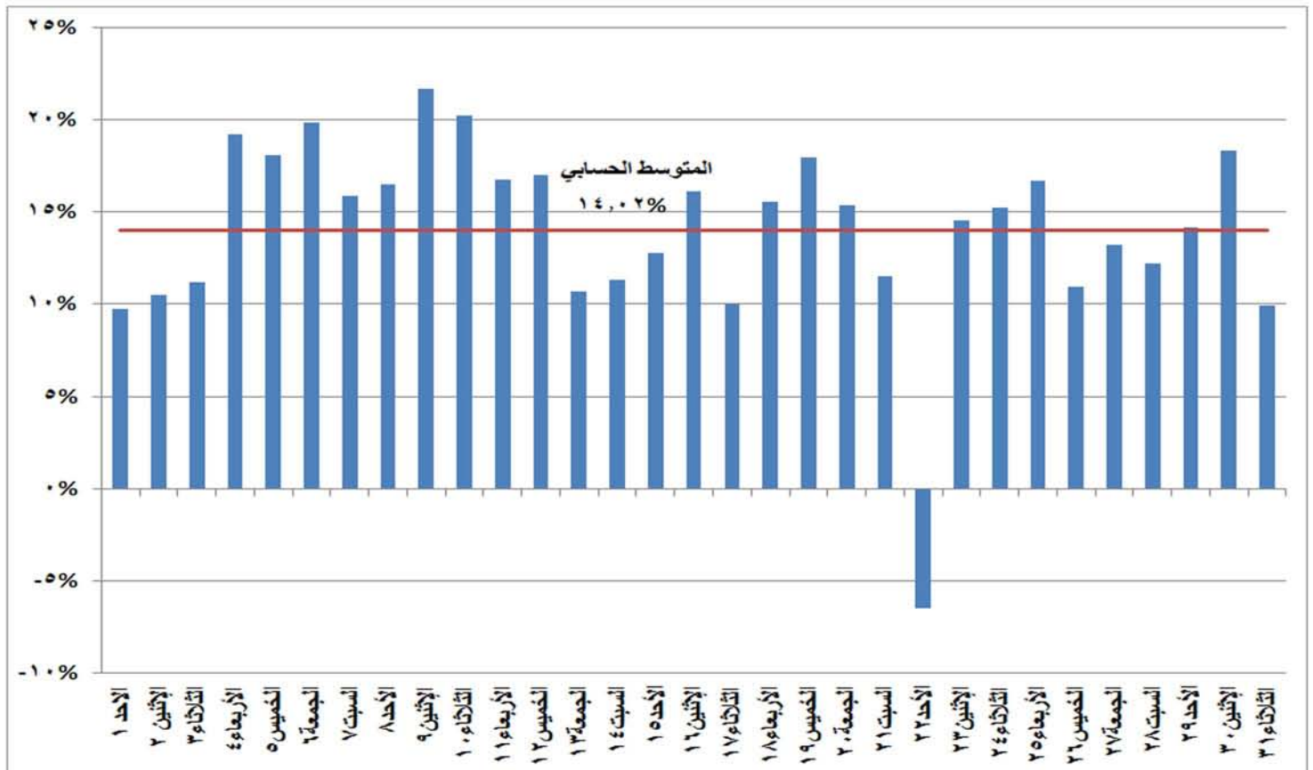
شكل (١٨) نسب التغير في استخدام الغاز الطبيعي في إنتاج الطاقة الكهربائية خلال شهر يوليو ٢٠١٨ مقارنة بالشهر المماثل من العام السابق
