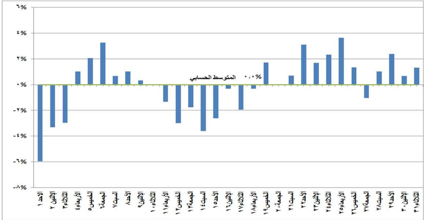
شكل (٩) النسب المئوية للتغير في الحمل الاقصى خلال شهر يوليو ٢٠١٨ مقارنة باليوم المماثل من العام الماضي
