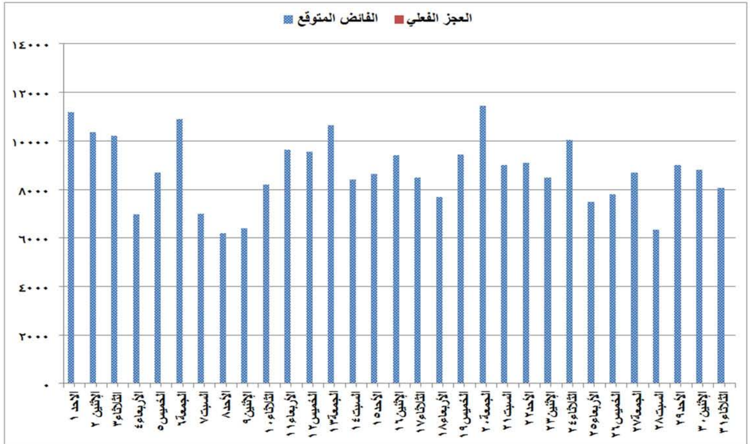
شكل (٧) الفااض والعجز المتوقع للقدرات خلال شهريوليو ٢٠١٨
